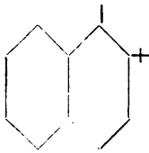
Schäffersche Säure. Schäffer. Annal. 152. 298.
